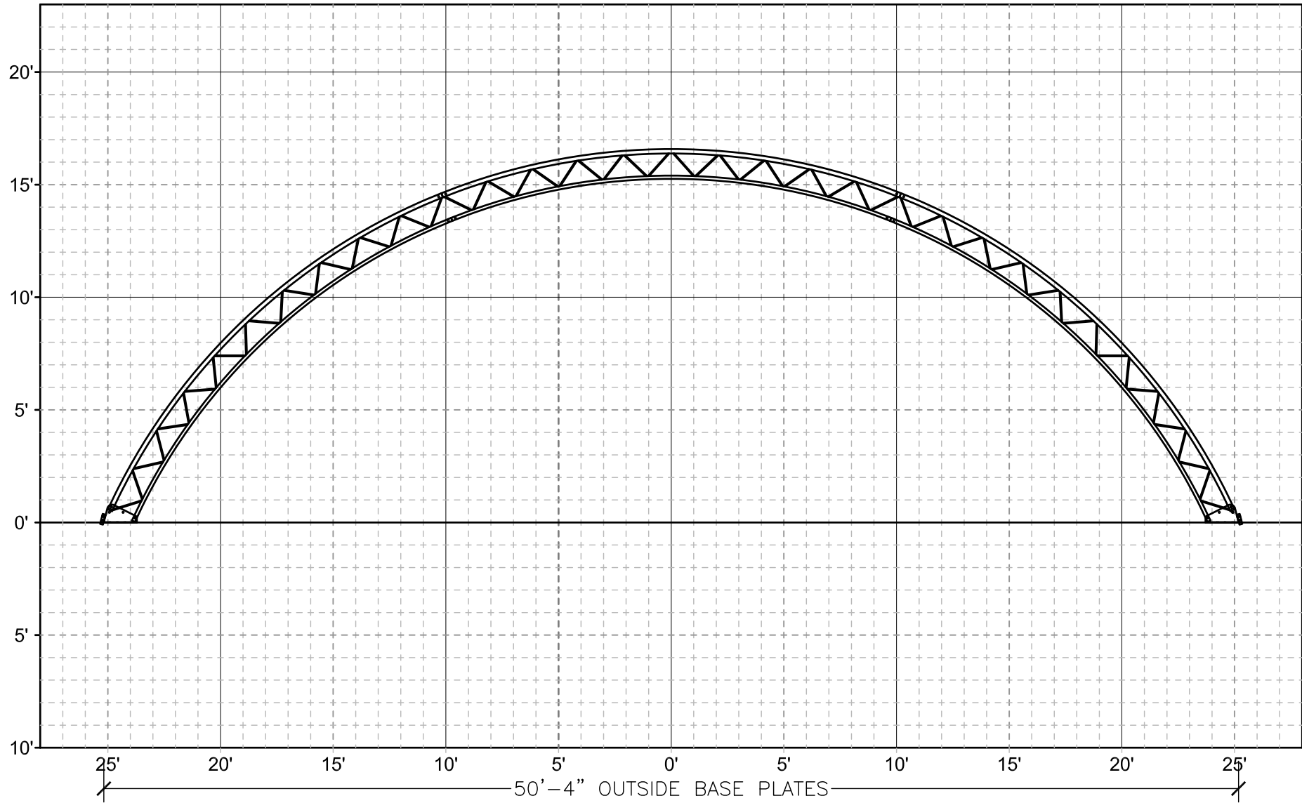
1'x1' GRID
